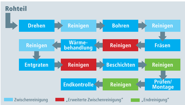
Abbildung 1: Beispiel einer Prozesskette (Quelle: SurTec Deutschland GmbH)
