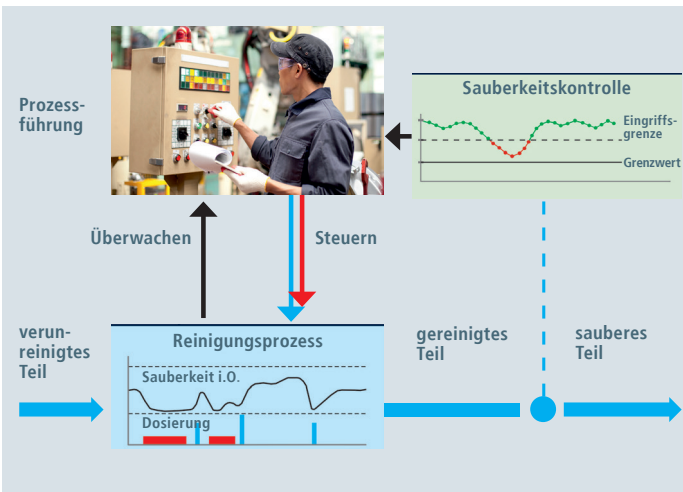
Abbildung 3: Überwachung qualitätsbeeinflussender Prozessparameter (Quelle: SITA Messtechnik GmbH)
